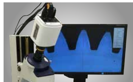
HDMI kamera a TM mikroszkóp okulárcsővére szerelve
